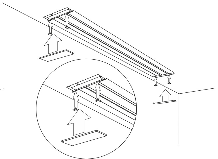
Rys.10 Mocowanie ekranu - faza 5 Montaż maskownic
