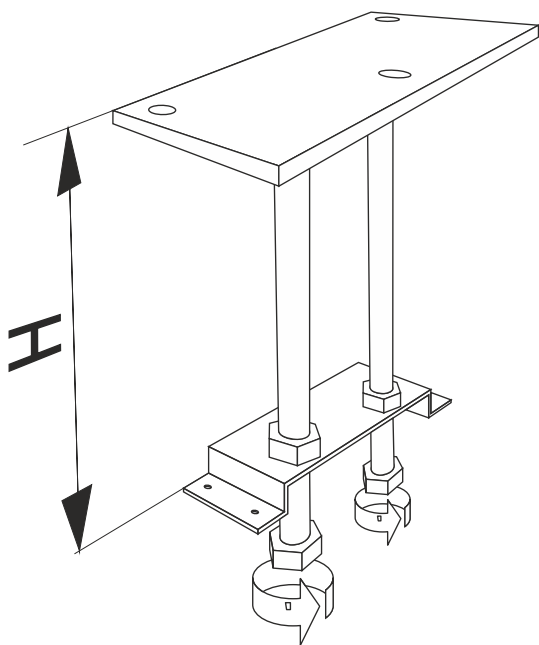
Rys.3 Przygotowanie szablonu do wyznaczania położenia podstawy mocowania
