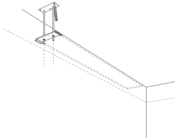
Rys.4 Wyznaczanie położenia otworów do instalacji mocowania sufitowego przy pomocy szablonu
